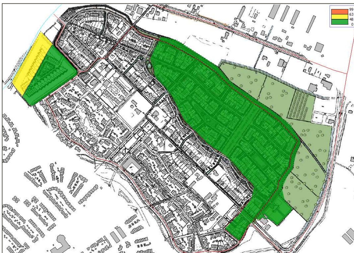
Afbeelding 6 Geluidcontouren (7,5 meter boven plaatselijk maaiveld) van de berekende geluidbelasting inclusief aftrek artikel 110g Wgh ten gevolge van de Zuiddreef
