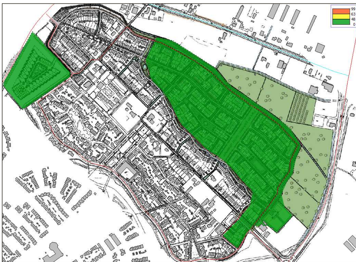
Afbeelding 5 Geluidcontouren (7,5 meter boven plaatselijk maaiveld) van de berekende geluidbelasting inclusief aftrek artikel 110g Wgh ten gevolge van de Oosterweg
