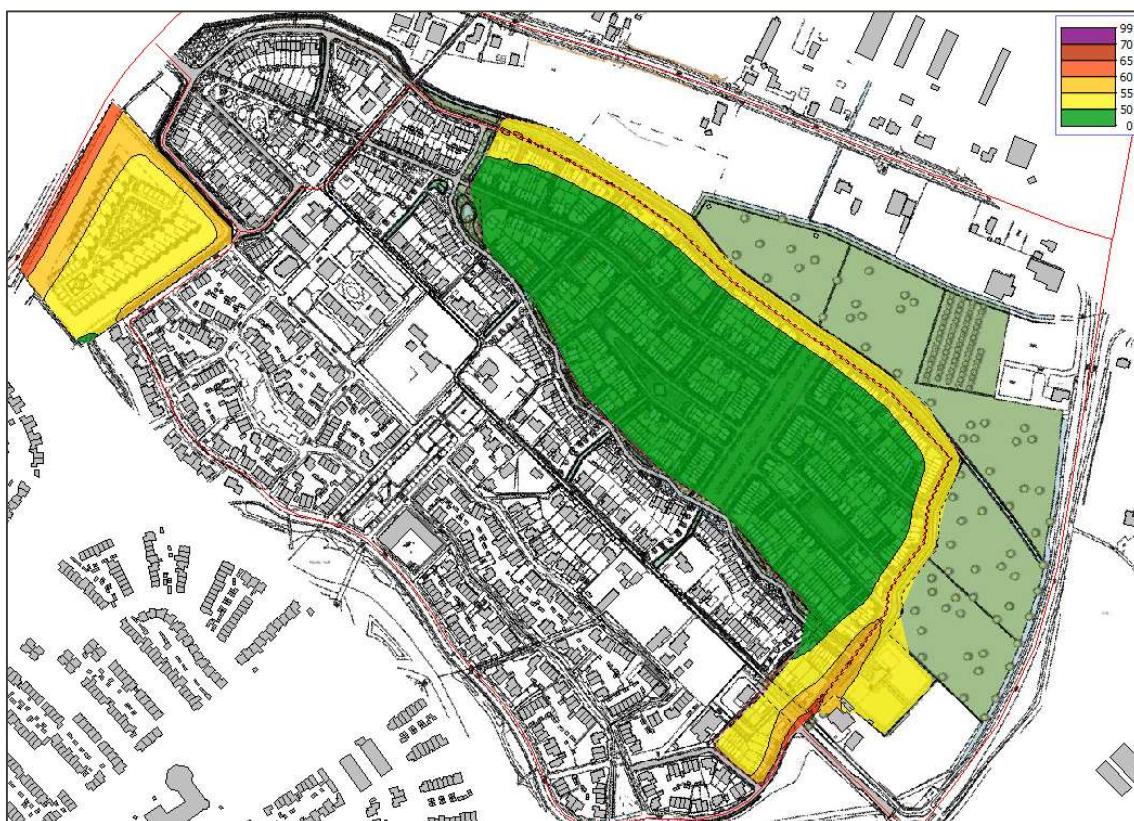
Afbeelding 10 Geluidcontouren gecumuleerde geluidbelasting (7,5 meter hoogte boven plaatselijk maaiveld) ten gevolge van alle wegen exclusief aftrek artikel 110g Wgh
