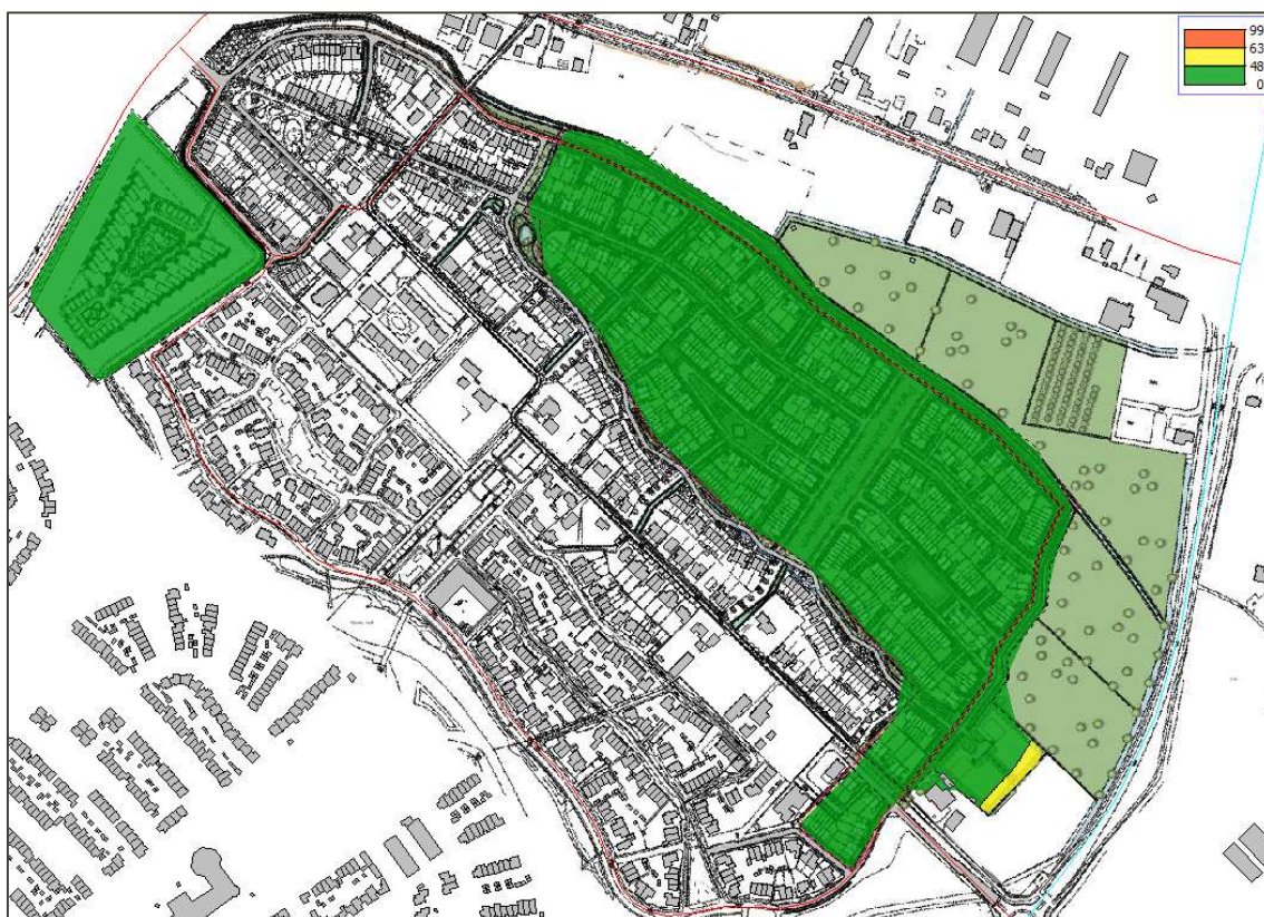
Afbeelding 4 Geluidcontouren (7,5 meter boven plaatselijk maaiveld) van de berekende geluidbelasting inclusief aftrek artikel 110g Wgh ten gevolge van de N324
