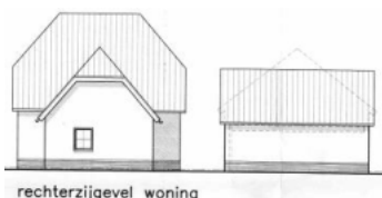
rechterzijgevel woning
