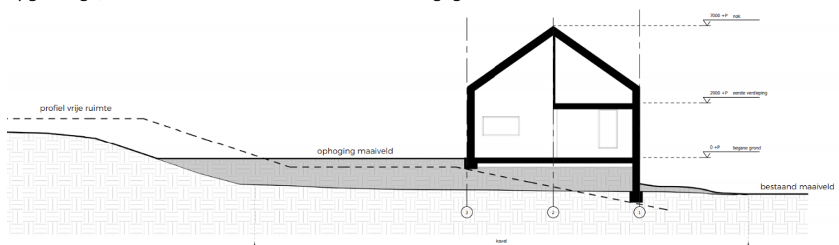
Afbeelding 6: Doorsnede woning inclusief profiel vrije ruimte
