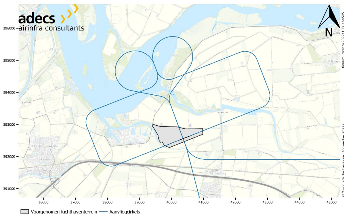
Figuur 12 Ligging van aanliegcirkels voor opstijgend en landend vliegverkeer.
