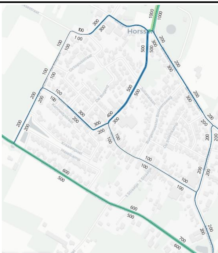
Etmaalintensiteiten
