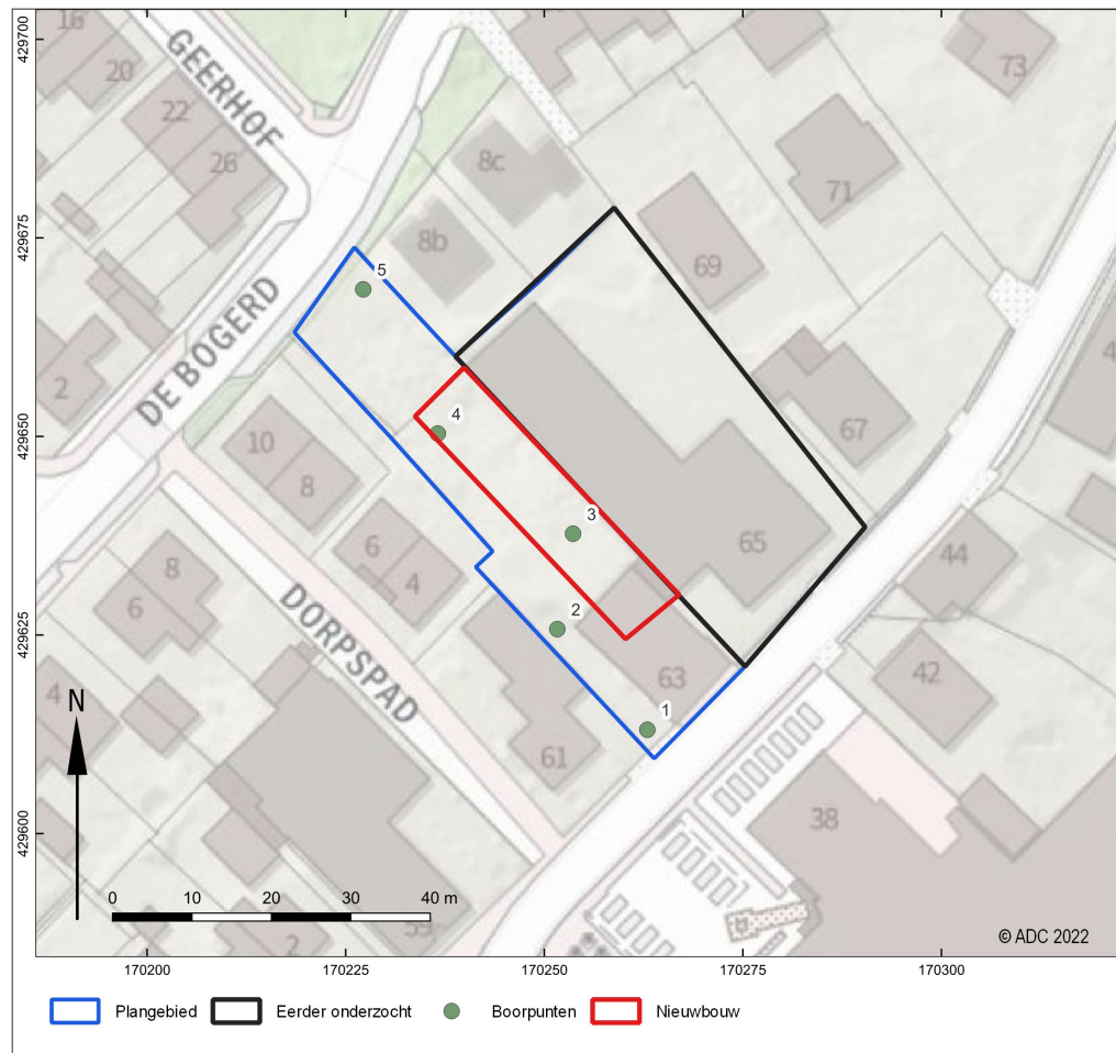
Afb. 14 Boorpuntenkaart
