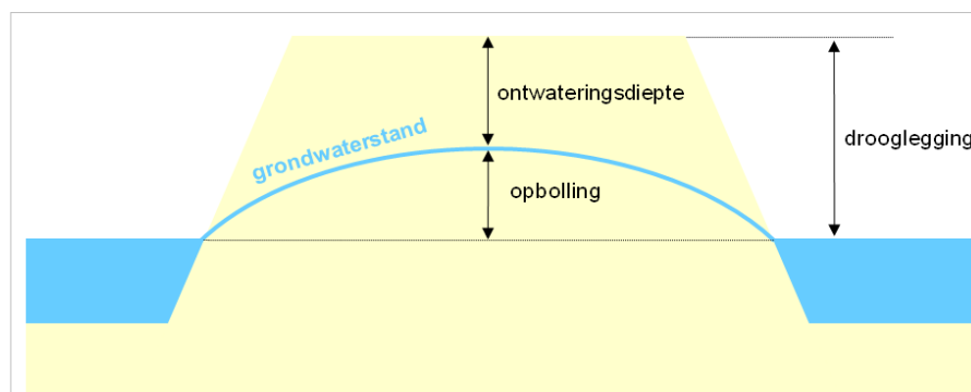
Afbeelding 11: Schematische weergave ontwateringsdiepte en drooglegging
