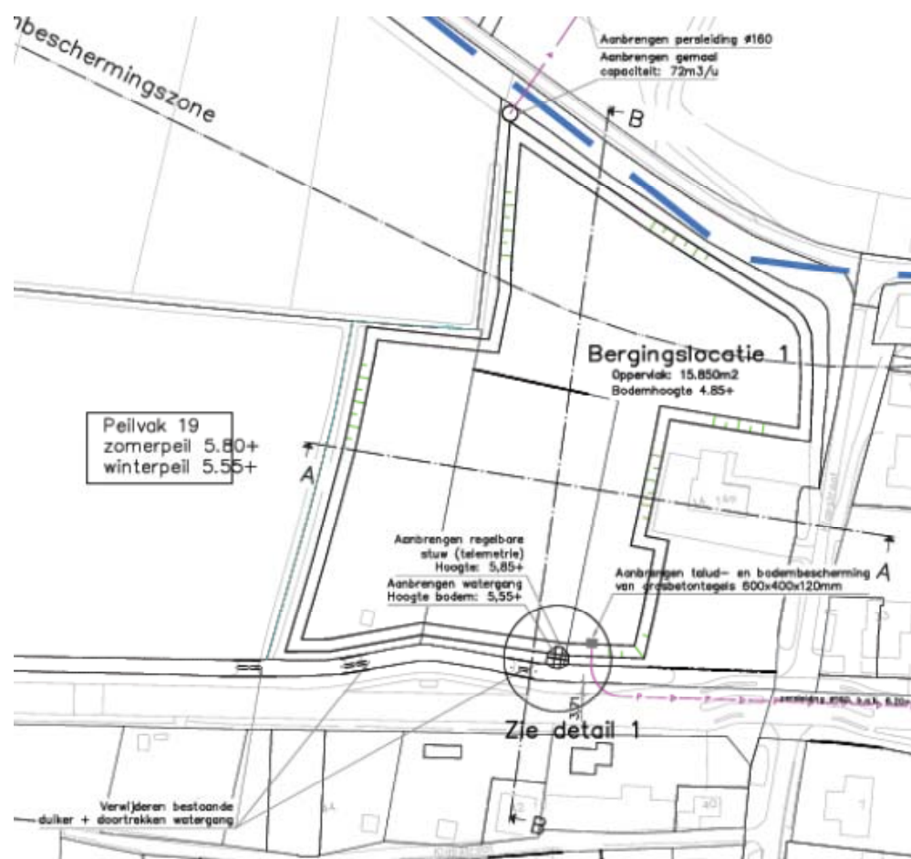
Figuur: Indicatieve inrichting kwelberging Klapstraat.
