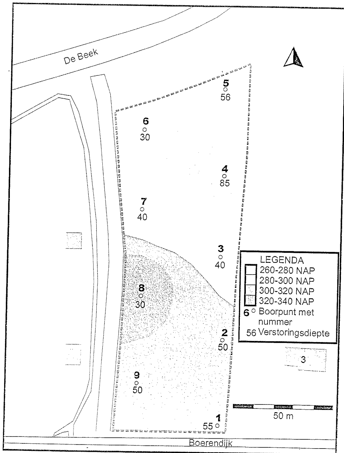
Figuur 4: Boorpuntenkaart Gieterveen, Boerendijk. De genummerde punten geven de uitgevoerde boringen weer. De nummers hiernaast geven de diepte aan tot waarop de bodem verstoord is. De kleuren geven de top van het dekzand t.o.v. NAP aan.
