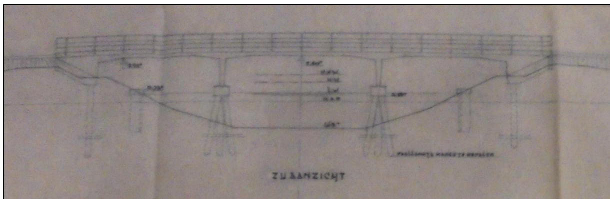
Figuur 8: Zijaanzicht van de te bouwen brug over de Oostermoerse Vaart.
