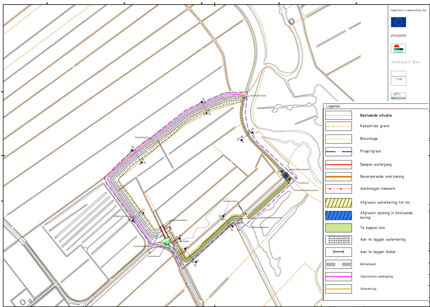
Figuur 1.2 Voorlopig ontwerp
