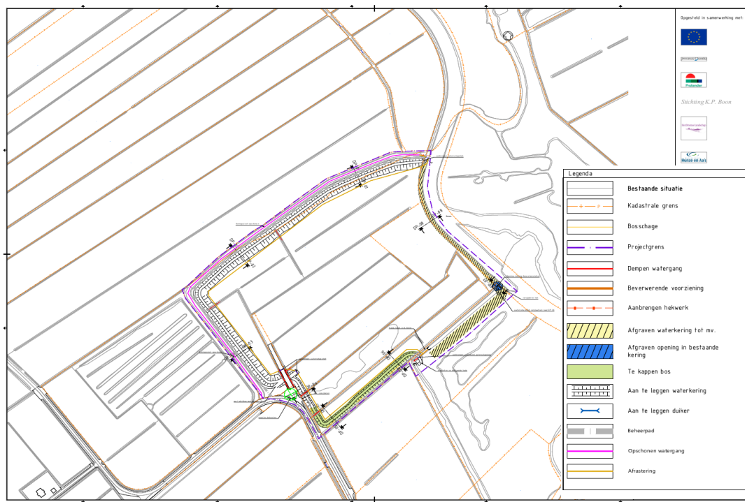
Figuur 1.2 Voorlopig ontwerp
