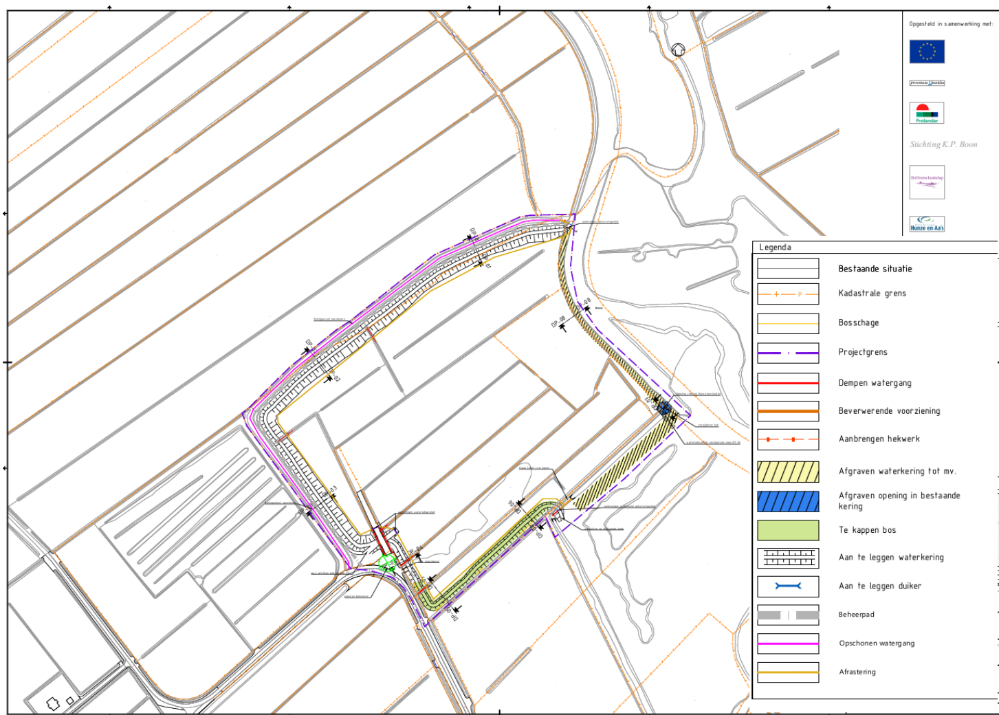
Figuur 2.3 Voorlopig ontwerp Boonspolder
