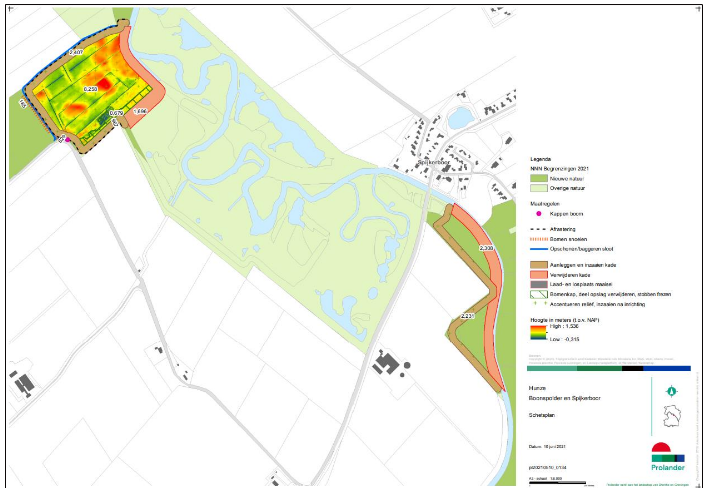
Figuur 2: Voorlopig Ontwerp Boonspolder en Bevergebied Spijkerboor (Prolander 2022).
