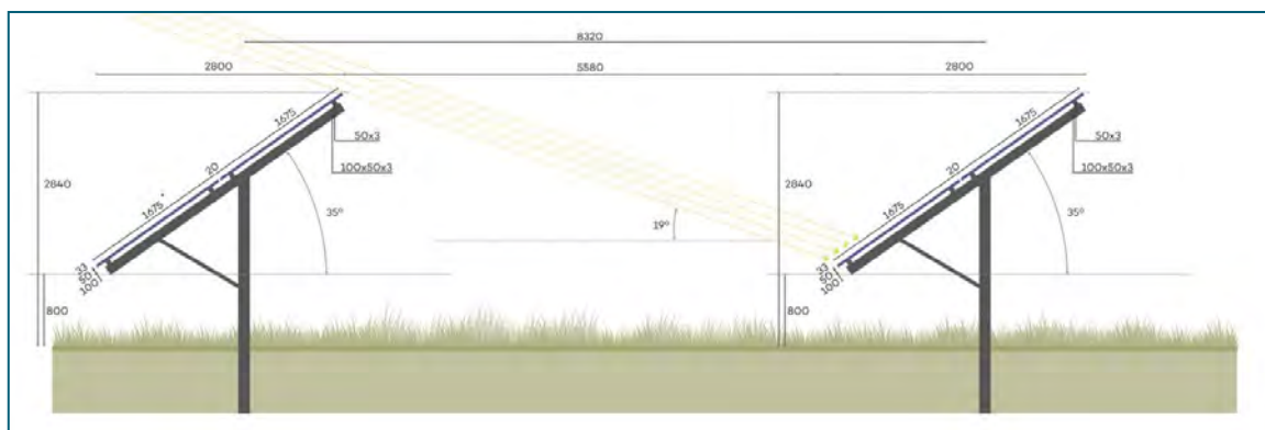
Afbeelding 4.3 Noord-zuidoriëntatie
