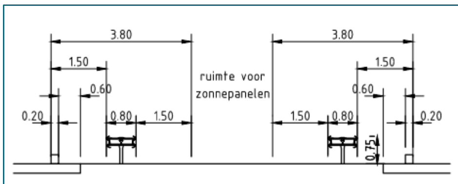
Afbeelding 4.11 Beschrijving middenberminrichting
