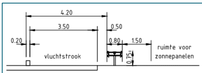
Afbeelding 4.10 Beschrijving buitenberminrichting
