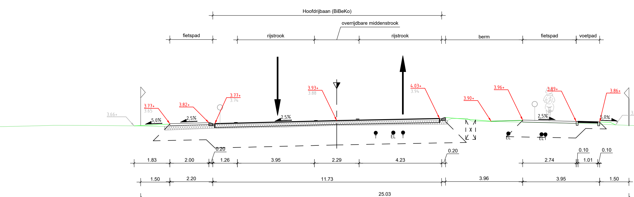
DOORSNEDE A SCHAAL 1 : 100 13.236
