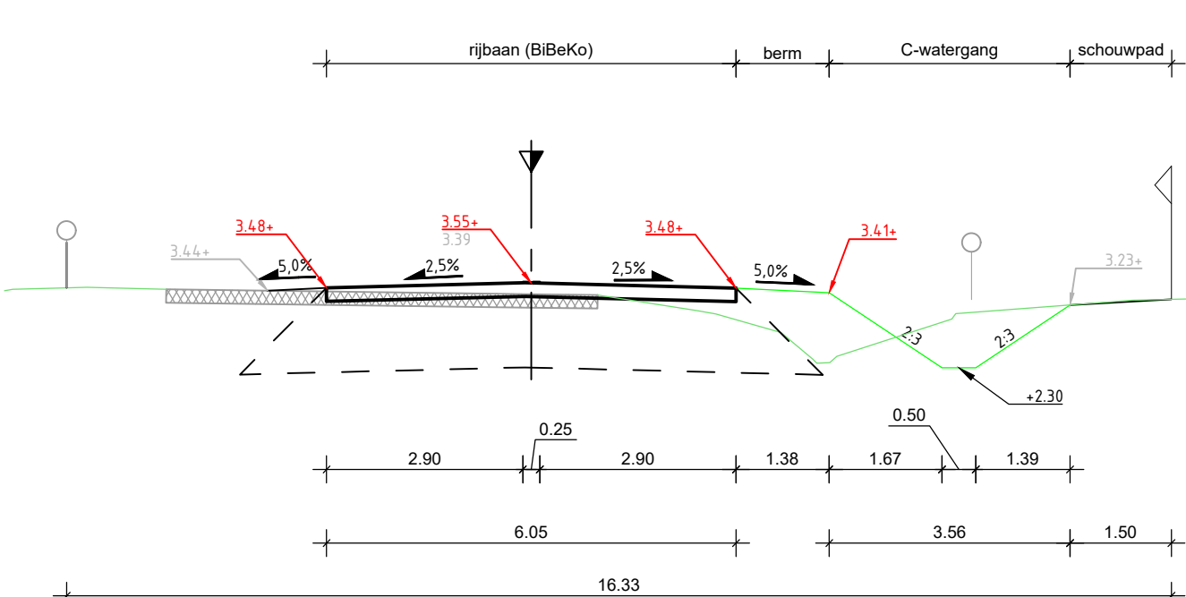
DOORSNEDE D SCHAAL 1 : 100 17 / 58
