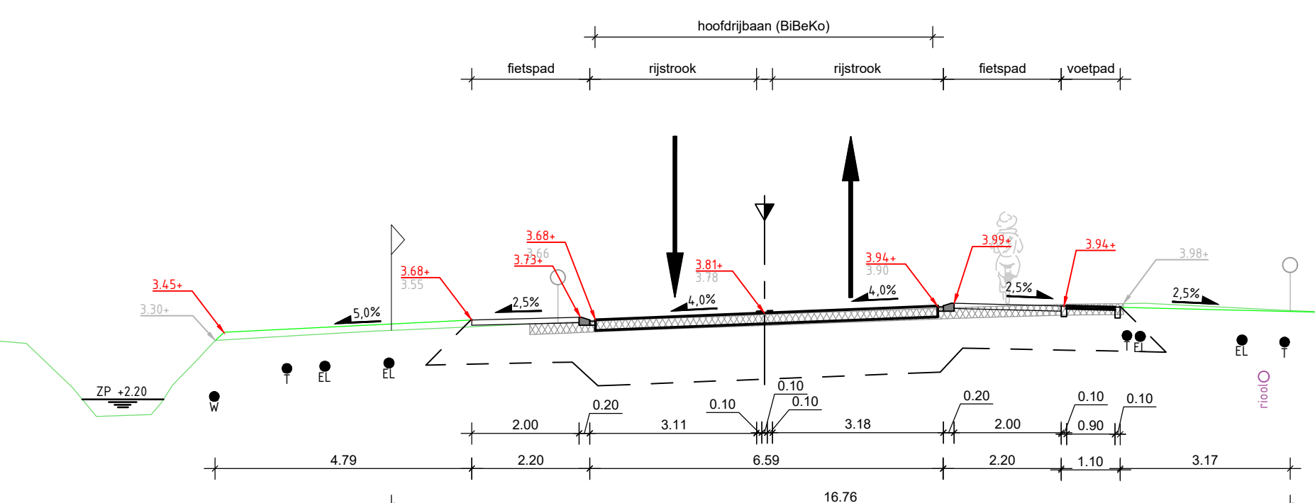
DOORSNEDE A SCHAAL 1 : 100 13.236
