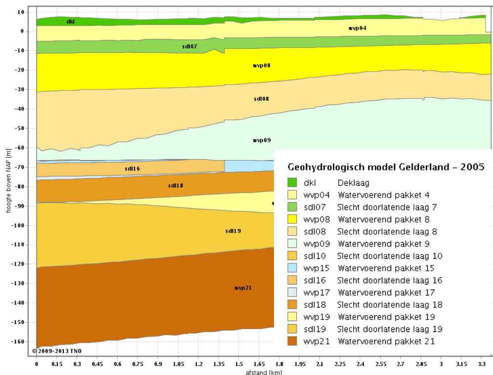
Figuur 3-1 Doorsnede geohydrologisch model REGIS II.0, TNO, DINO-Loket
