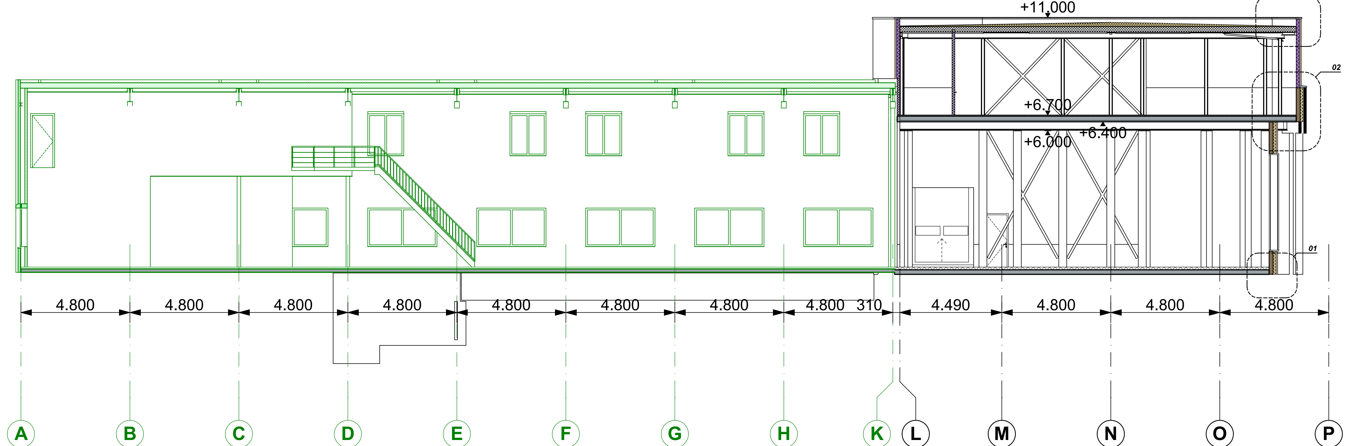
Doorsnede A1
