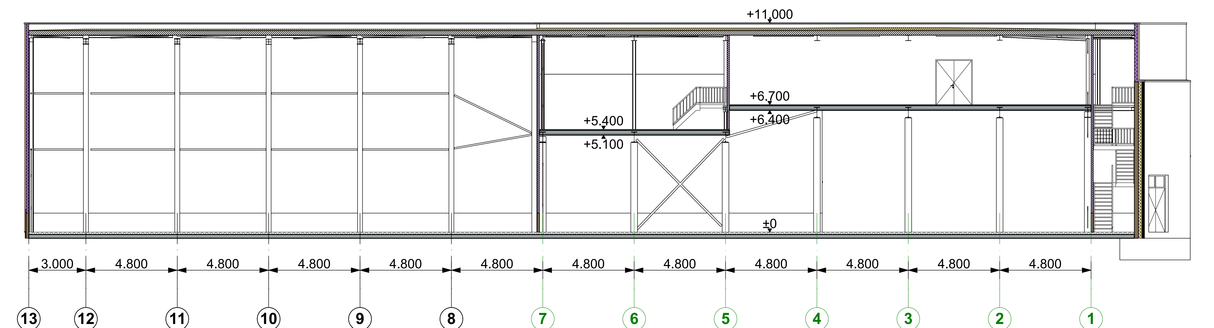
1:100 Doorsnede B3 Te Bouwen
