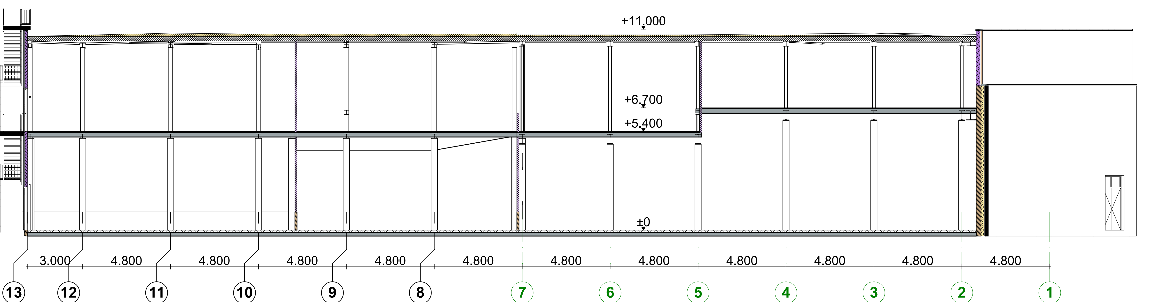
1:100 Doorsnede B4 Te Bouwen
