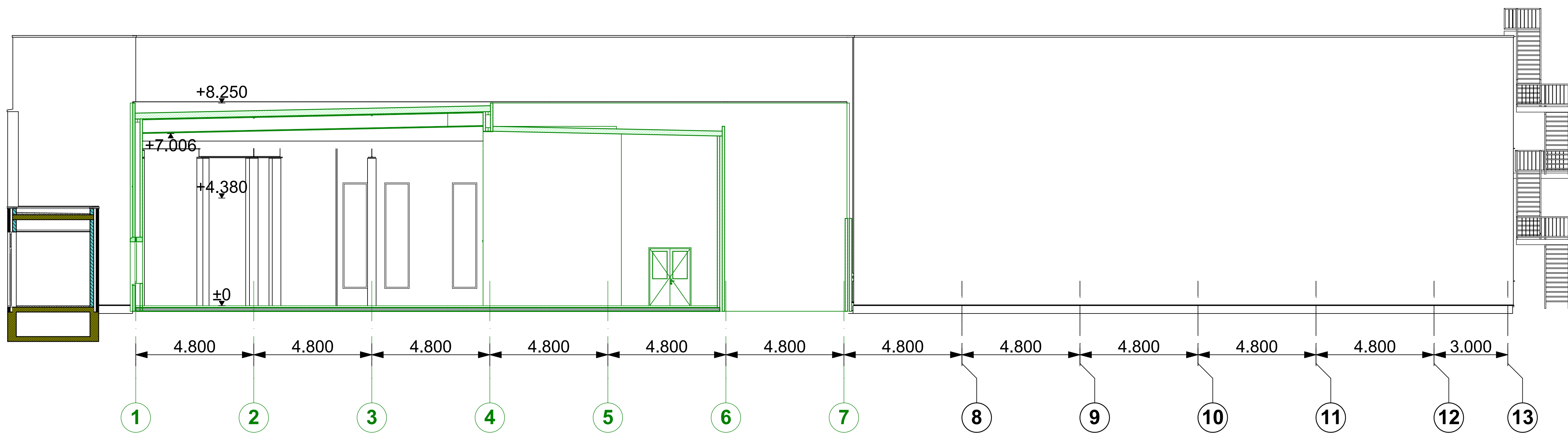
1:100 Doorsnede B1 Te Bouwen
