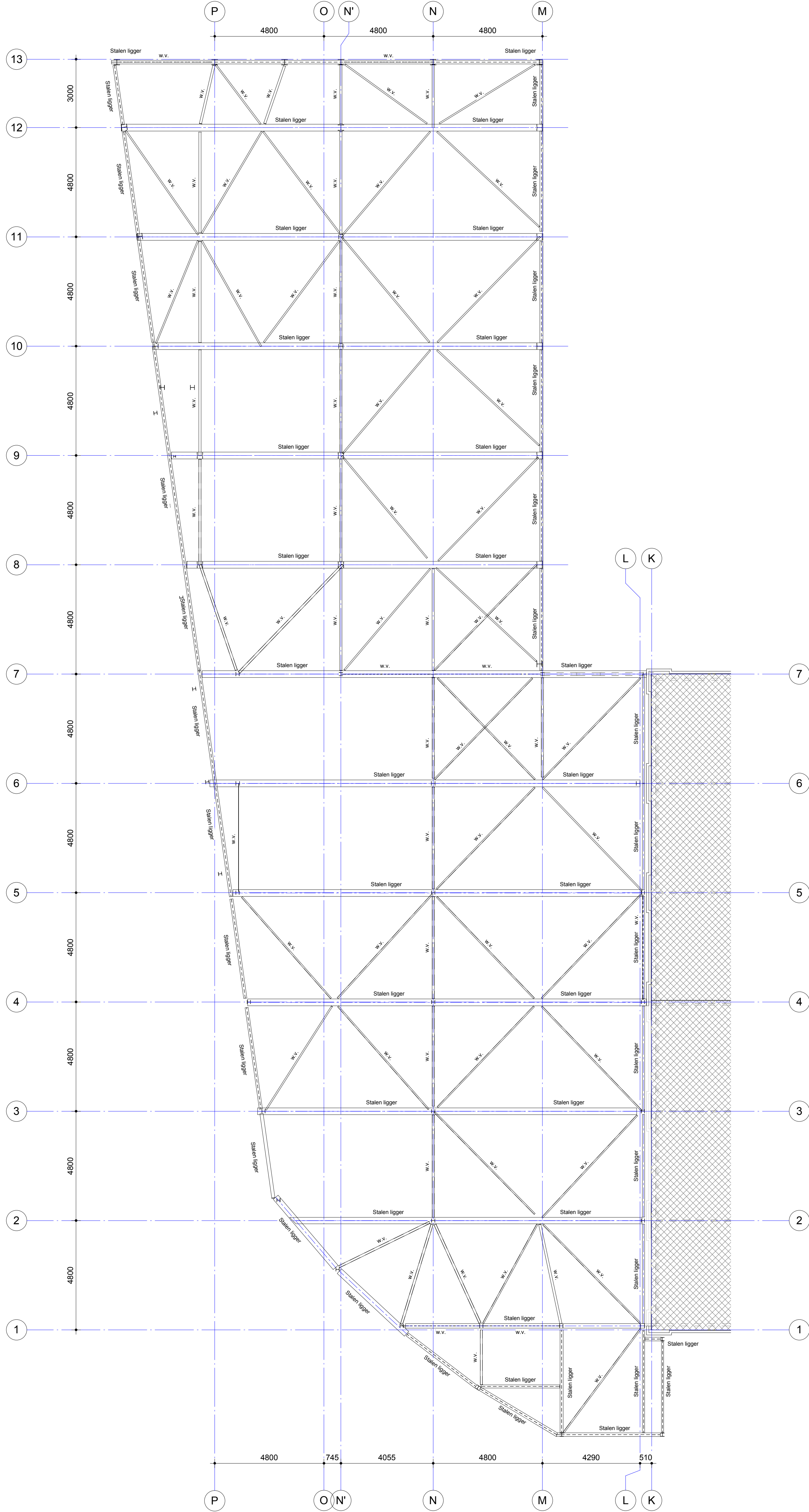
Overzicht dak
