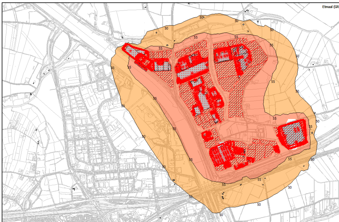
Figuur 7: Combinatiemodel Medel (geoptimaliseerd) inclusief uitbreiding Medel fase 1 en 1a.
