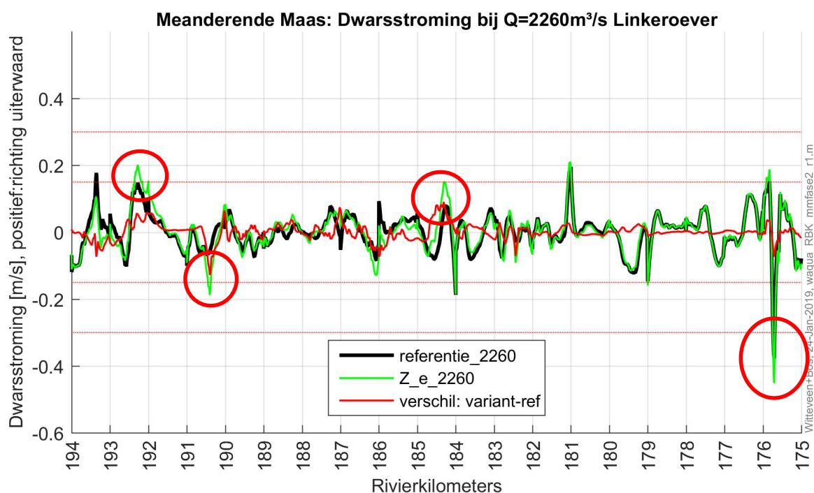
Afbeelding 7.11 Dwarsstroming op de linker bakenlijn voor alternatief Z, de referentie en verschillen hiertussen bij 2260 m 3 /s (in onderstaand afbeelding heet Z 'Z_e' in verband met modelopzet)
