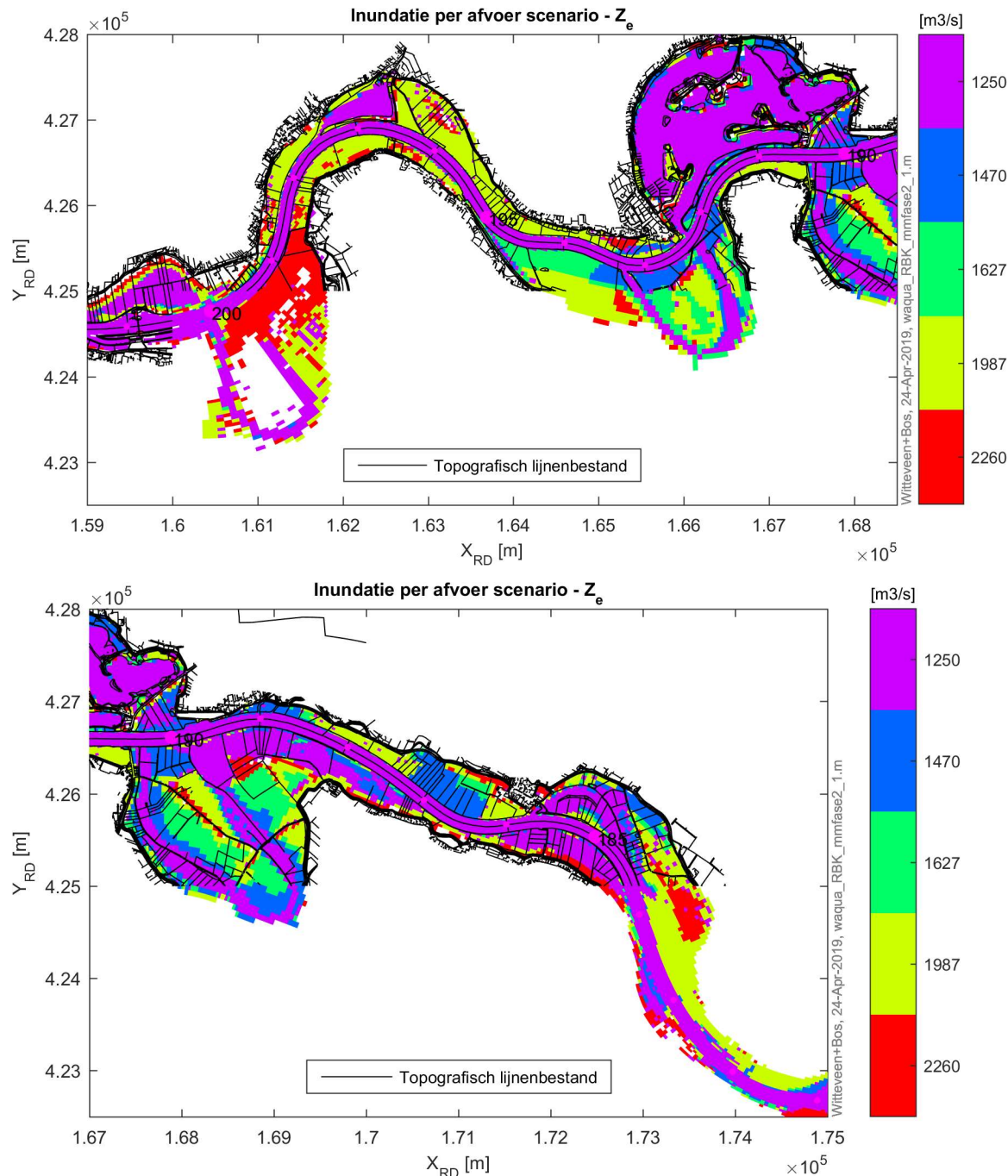
Abbeelding 7.3 Inundatiekaart alternatief Z (boven: west, onder: oost) (zie Tabel 7.11 voor legenda uitleg)
