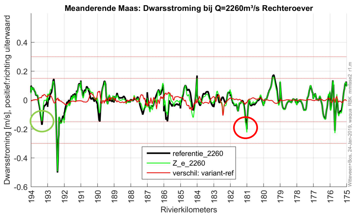
Afbeelding 7.10 Dwarsstroming op de rechterbakenlijn voor alternatief Z, de referentie en verschillen hiertussen bij 2260 m 3 /s (in onderstaand afbeelding heet Z 'Z_e' in verband met modelopzet)
