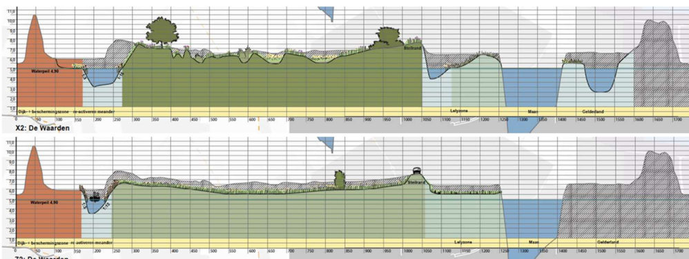
Afbeelding 7.18 Doorsneden van de Waarden. X (boven) reliëf versterkt afgegraven, Z (beneden) reliëf afgevlakt
