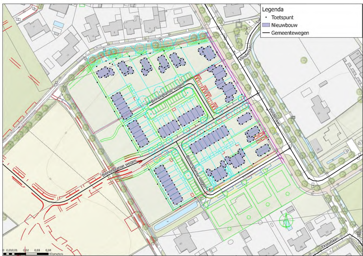
Figuur 3.1 Detailoverzicht van Fazantlaan-Oost met geprojecteerde nieuwbouw en toetspunten waar geluid is berekend.
