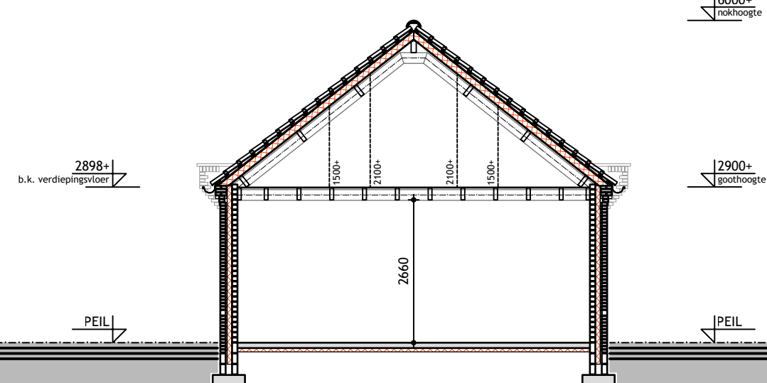
DOORSNEDE bijgebouw
