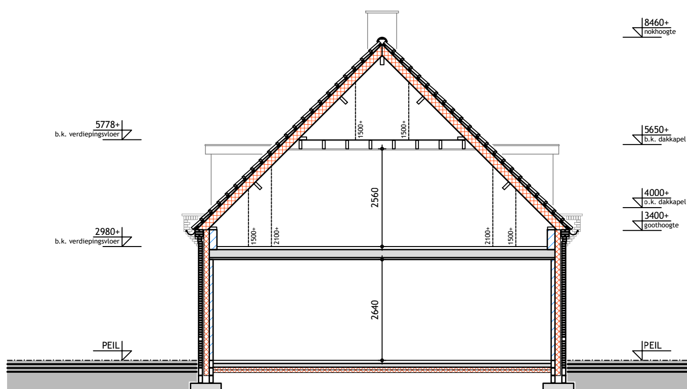
DOORSNEDE woonhuis
