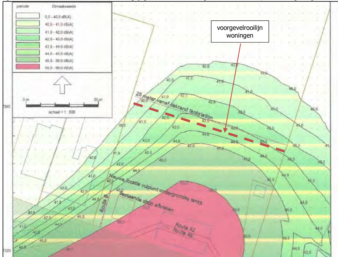
Figuur 7.3: Geluidcontouren etmaalwaarde langtijdgemiddeld beoordelingsniveau tankstation, beoordelingshoogte 5 m
