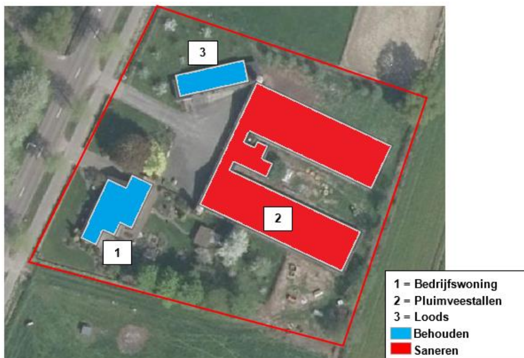
• Afbeelding 2: situatieschets van de inrichting (bron: Reland ontvangen op 18-12-2019)
