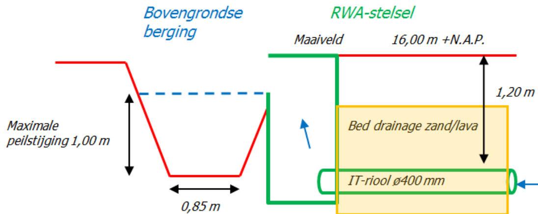
Principe IT-rigol met grindkoffer en bovengrondse berging
