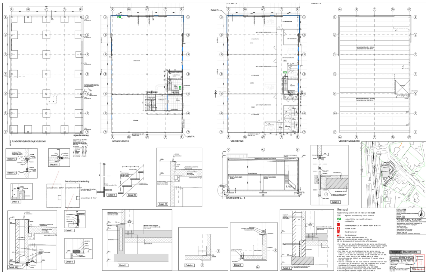
Uitsnede bouwtekening
