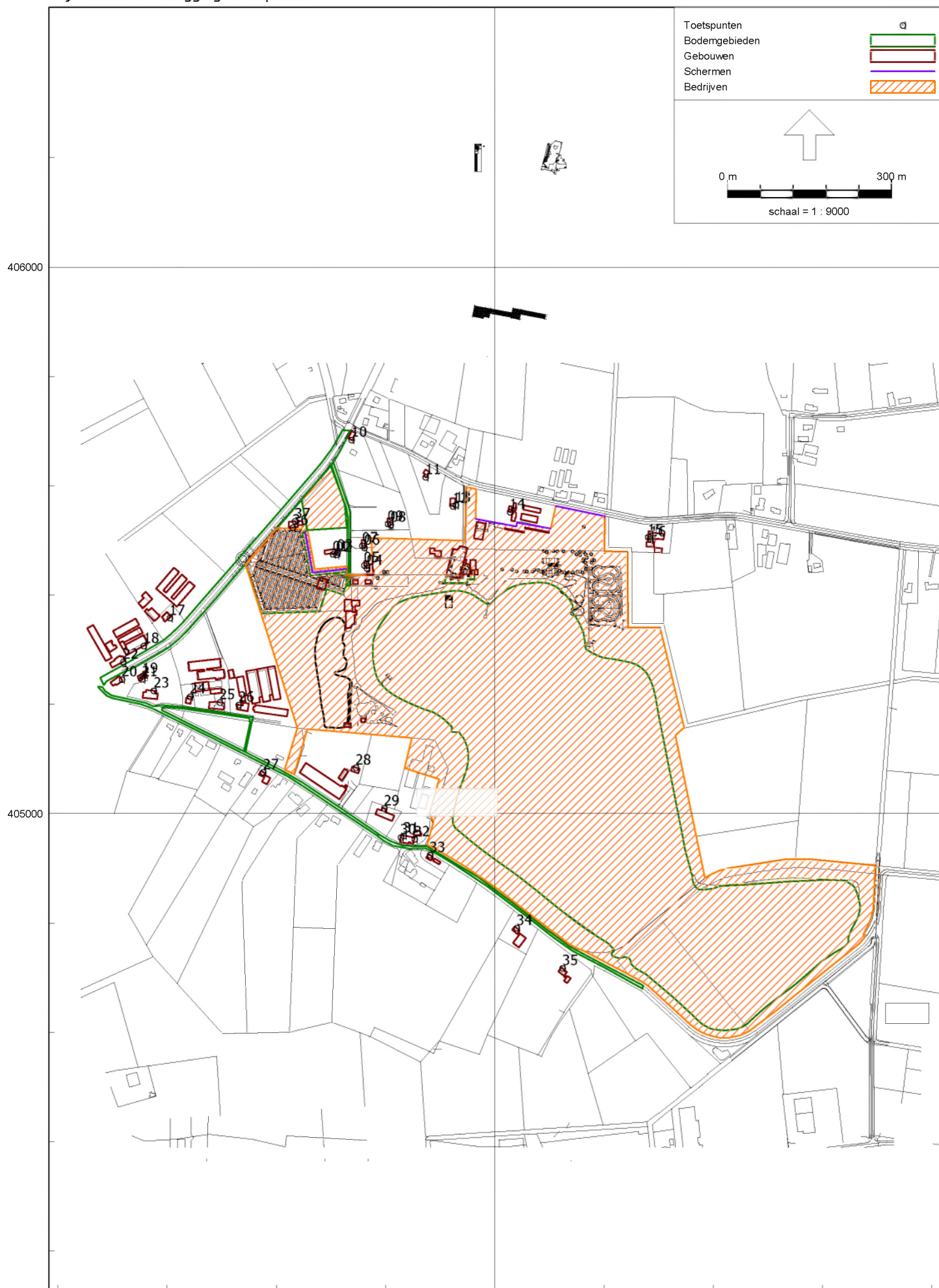
Figuur 1 Plaatselijke situatie met ligging rekenpunten
