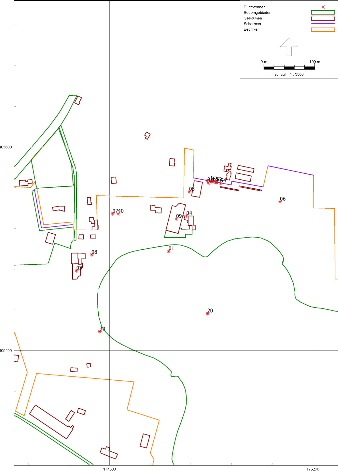
Figuur 7 Ligging puntbronnen LAr,LT
