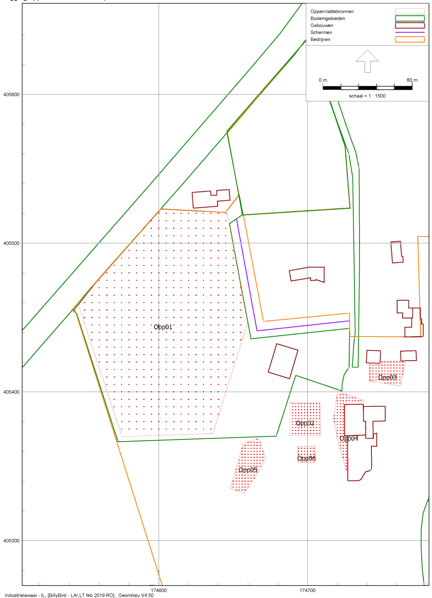
Figuur 11 Ligging oppervlaktebronnen LAr,LT
