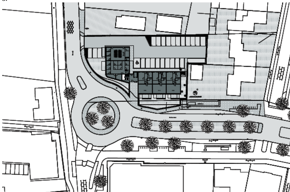
Figuur 2. Tekening van de toekomstige situatie.
