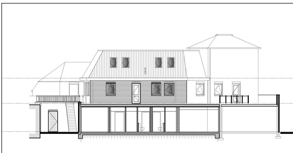
Afbeelding 9: linker zijgevel van de beoogde ontwikkeling
