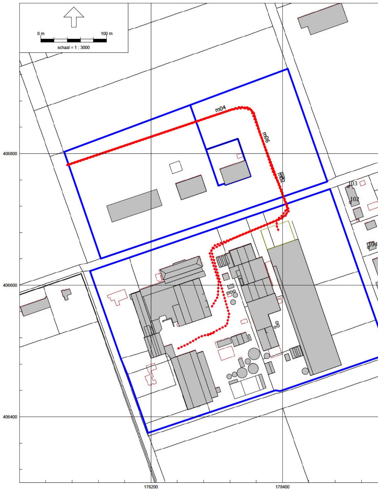
figuur 5j: Overzicht rekenmodel met positie geluidbronnen
