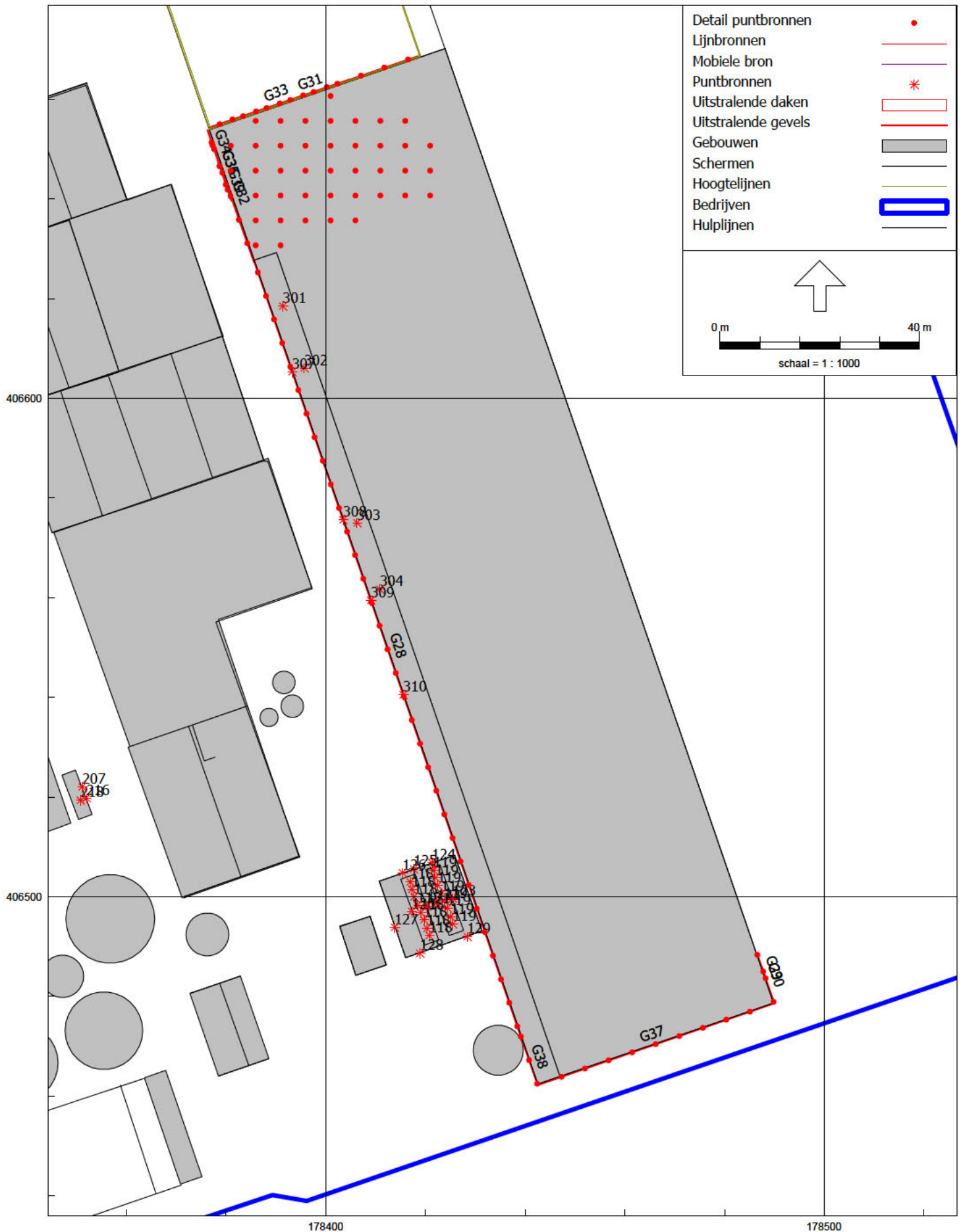
figuur 5a: Overzicht rekenmodel met positie geluidbronnen
