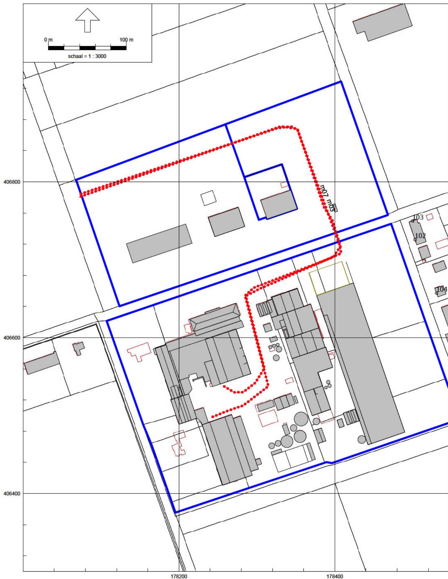
figuur 5k: Overzicht rekenmodel met positie geluidbronnen
