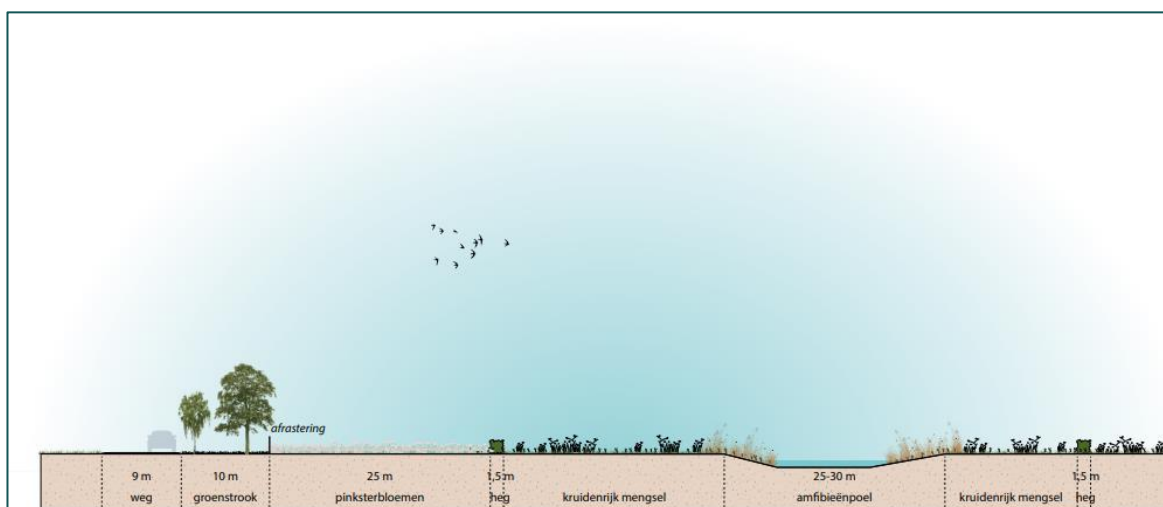
Figuur 3.2 Een dwarsprofiel van de inrichting zoals weergegeven in figuur 3 en betreft de percelen k559, k1247, k1249, k1251 en k1253. In bijlage I is een grotere weergave toegevoegd.
