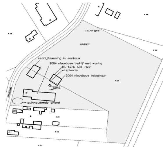
Figuur 4: Uitsnede situatietekening 8a (Archimil, 2006).
