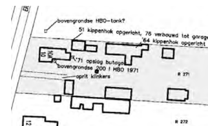
Figuur 5: Uitsnede situatietekening 10-10a (Archimil, 2006).
