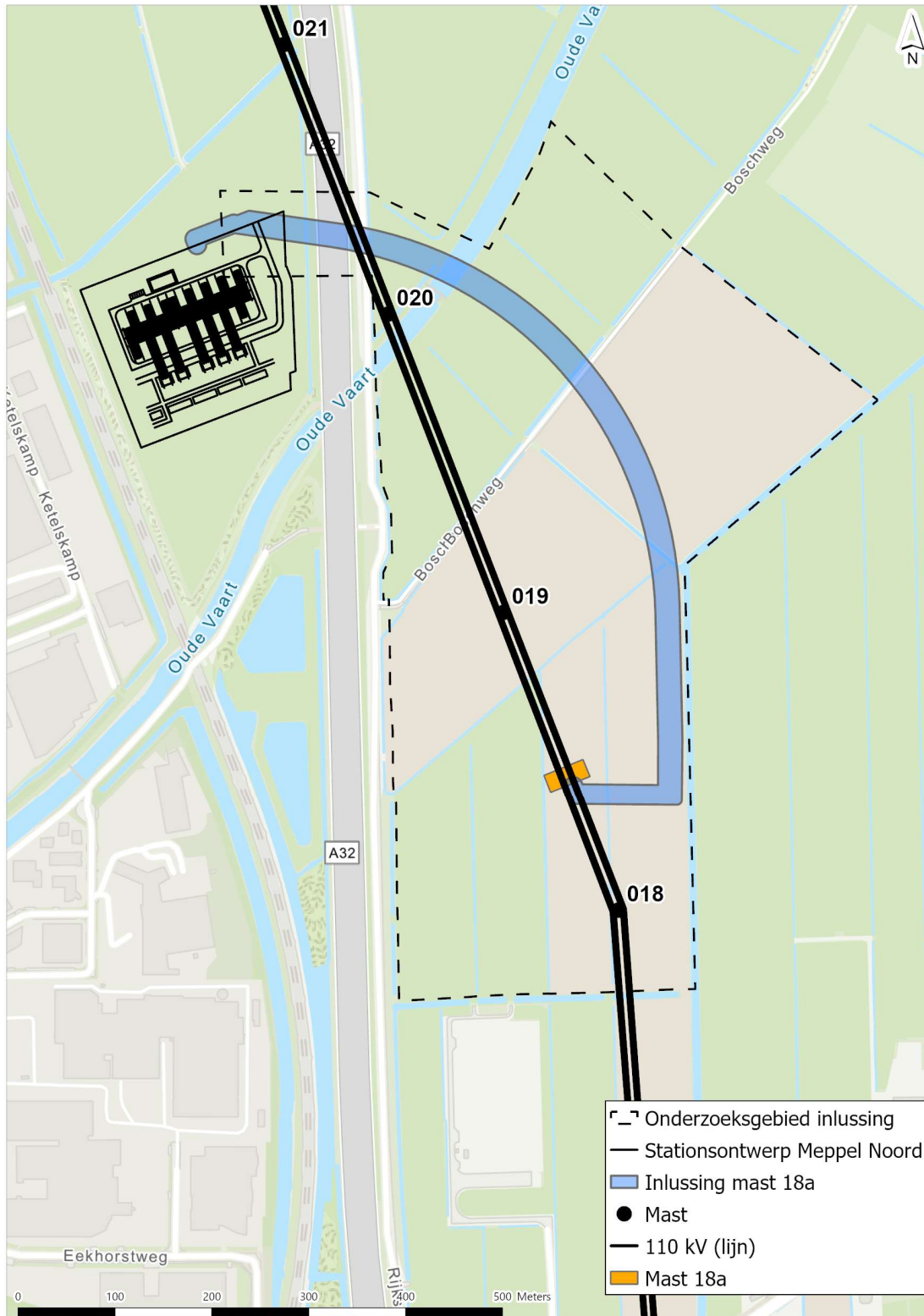
Afbeelding 2.3 Overzichtskaart beoogde situatie, met in blauw de nieuwe ondergrondse kabelverbinding, en in oranje het opstijgpunt
