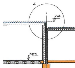
DOORSNEDE T. P. V. ERFGRENS
