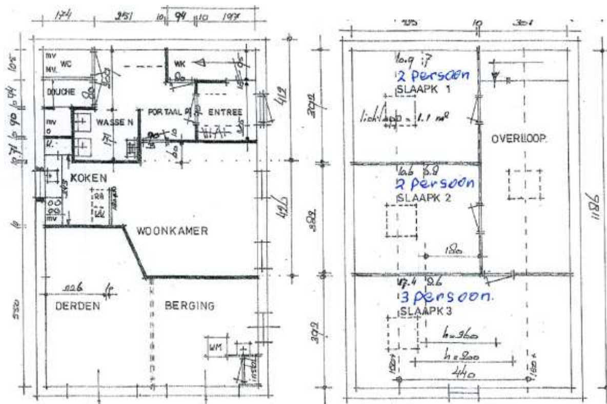
Figuur 6 c. Bouwtekening huisvesting 7 arbeidskrachten, garage begane grond (links) en verdieping (rechts)
