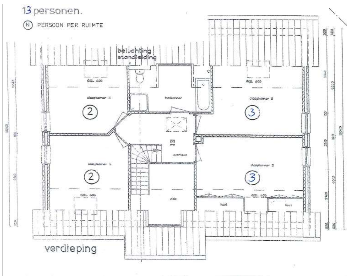
Figuur 6 b. Bouwtekening huisvesting 13 arbeidskrachten, woning verdieping
