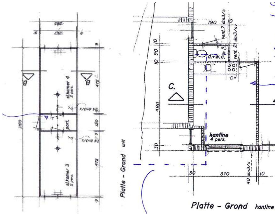
Figuur 6. Bouwtekening huisvesting van 4 arbeidskrachten.
