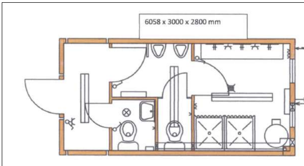
Figuur 6b. Tekening sanitairunit
