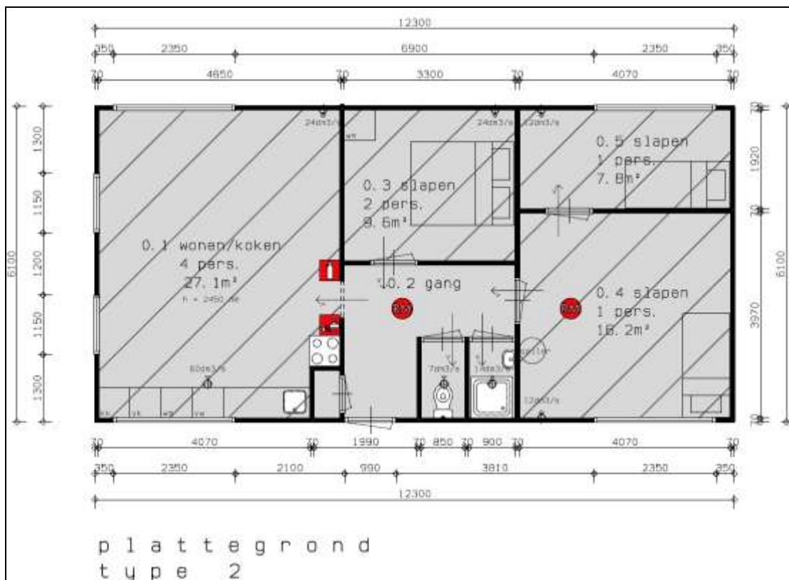
Figuur 6. Bouwtekening huisvesting
