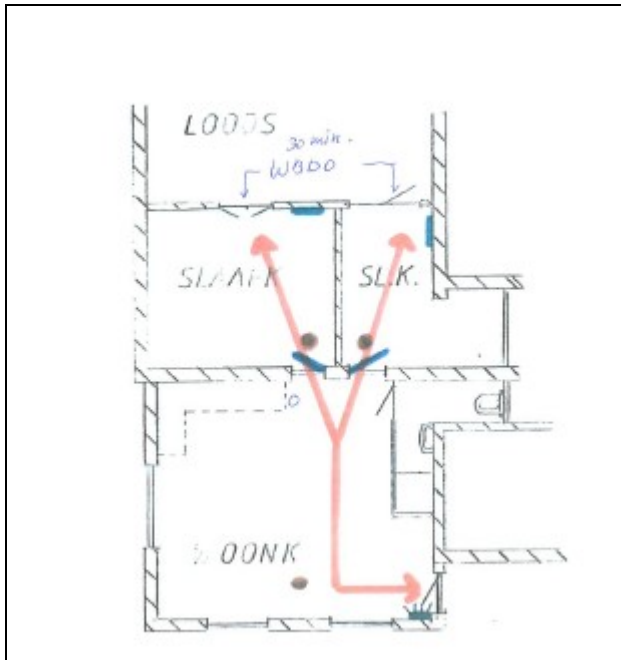
Figuur 6. Bouwtekening huisvesting 6 arbeidskrachten
