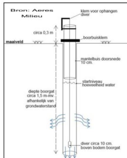
Afbeelding 7: Principetekening Porchetttest
