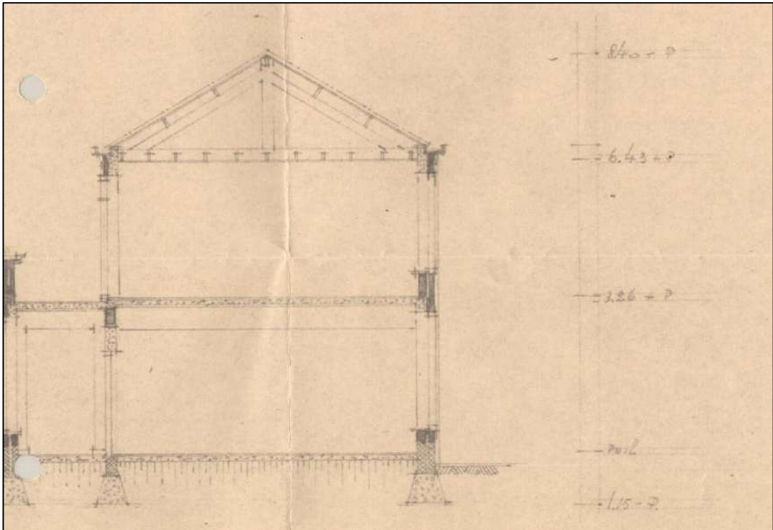
Afbeelding 17: Uitsnede bouwtekening ketelhuis d.d. 1954 (BHIC toeg. nr. 1478 en inv. nr. 1954.0015).
