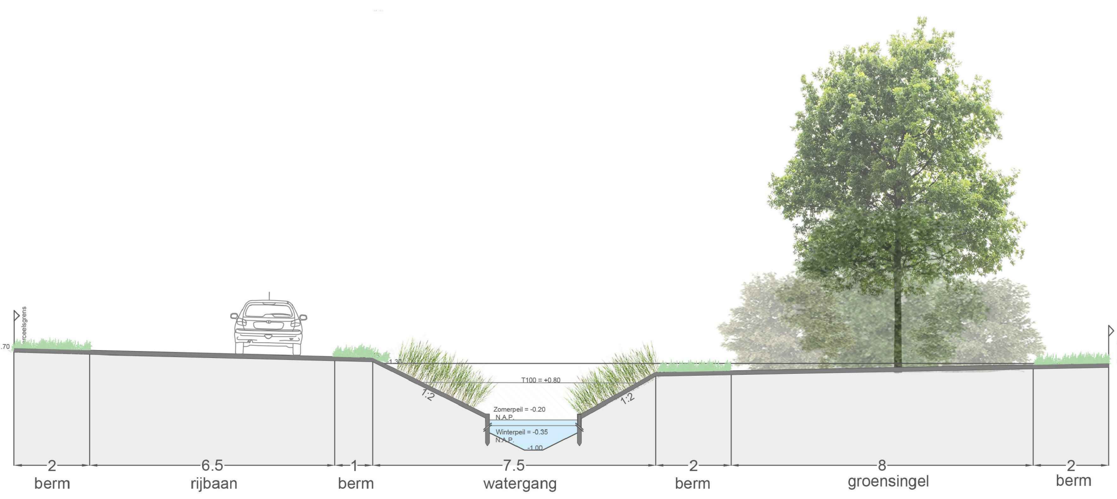
Profiel C-C
