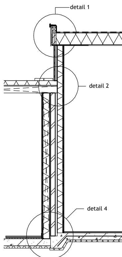
Doorsnede D-D
