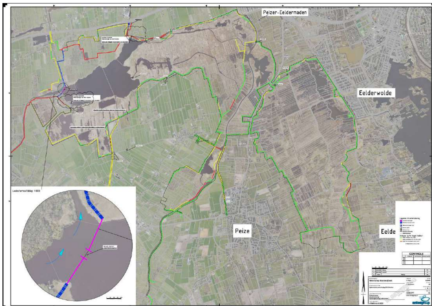
Figuur 1.1: Schematisch overzicht van de benodigde wijzigingen aan de kades. In rood zijn de kades met ruim onvoldoende hoogte, geel de kades met onvoldoende hoogte en groen de kades met voldoende hoogte.
