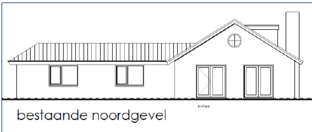
Bestaande noordgevel woning Achterloseweg 41
