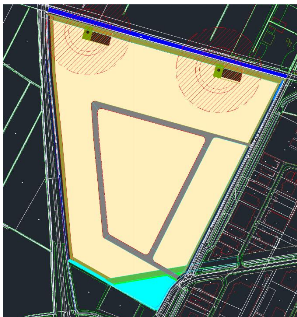
Figuur 1: planschets
