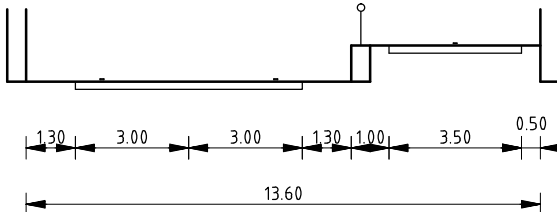
Principe dwarsprofiel (Tunnelbak) Schaal 1:200
