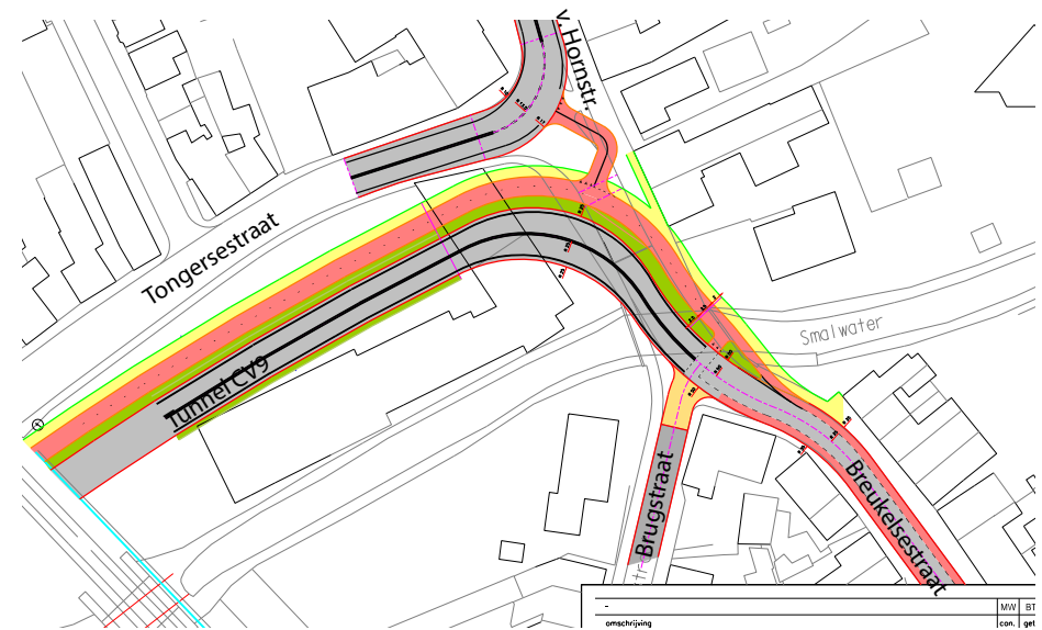
Schetsontwerp oostelijke toerit tunnelvarianten CV9
