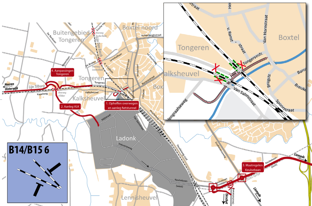
Overzichtskartaal B14/B15 Variant 6: Omleiding Zuidelijke Randweg (beide overwegen gesloten)
