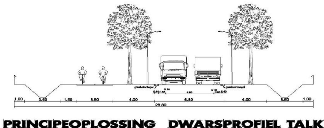
Figuur 2.2: Dwarsdoorsnede nieuwe verbindingsweg
