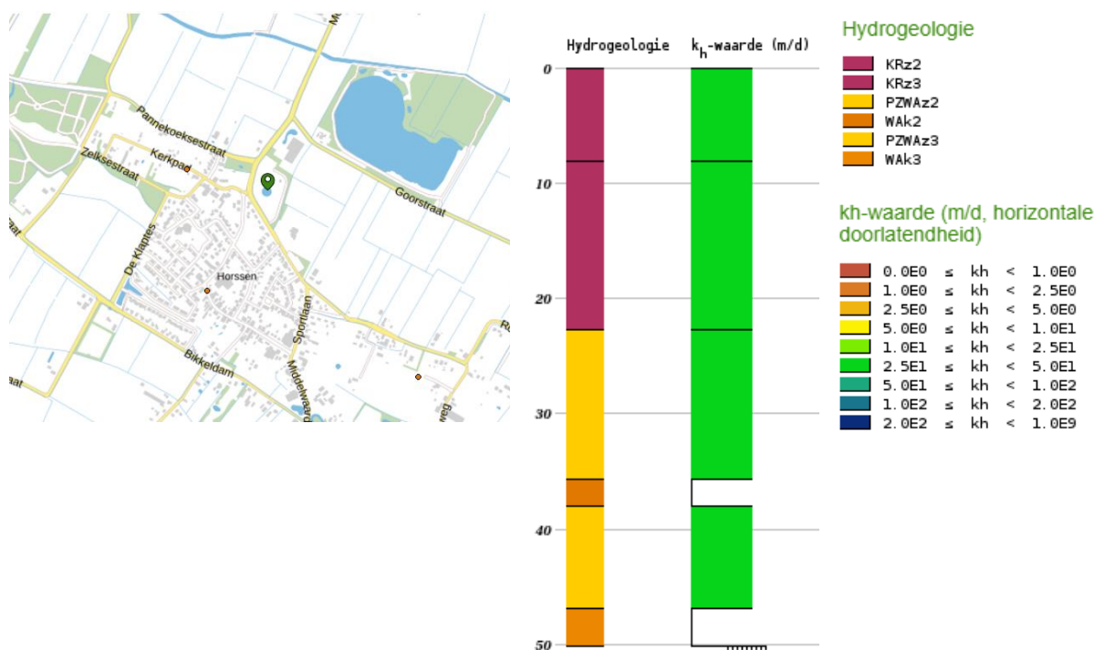
Figuur 4 Geohydrologisch model gebaseerd op REGIS II (bron: DinoLoket)
