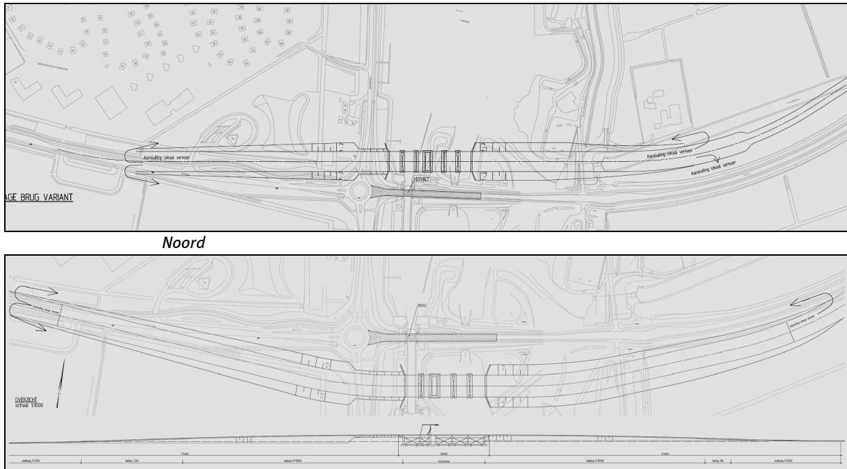
Figuur 16.3 Schetsontwerpen lage brug [DHV, 2008-2009]
