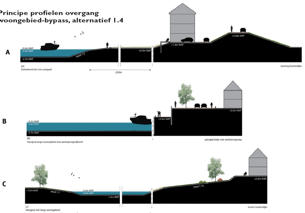
Figuur 3.9 Doorsnedes overgang woongebied-bypass alternatief 1.4 [H+N+S, 2009]
