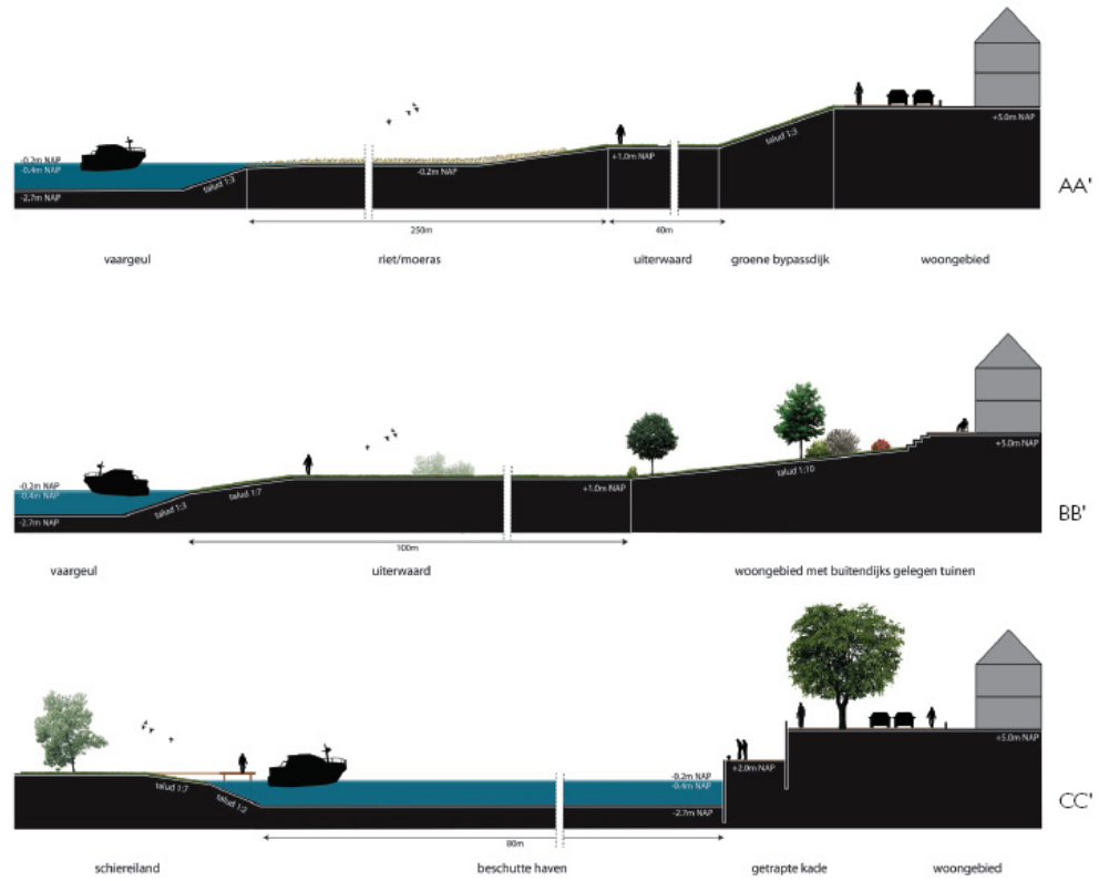
Figuur 21.5 Doorsnede woongebied voorkeursalternatief [H+S+N, 2009]
