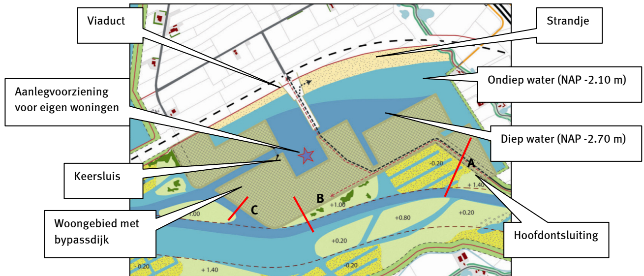
Figuur 3.6 Uitsnede woongebied alternatief 1.2 (zie figuur 3.5 voor doorsnede A, B en C) [H+N+S, 2009]
