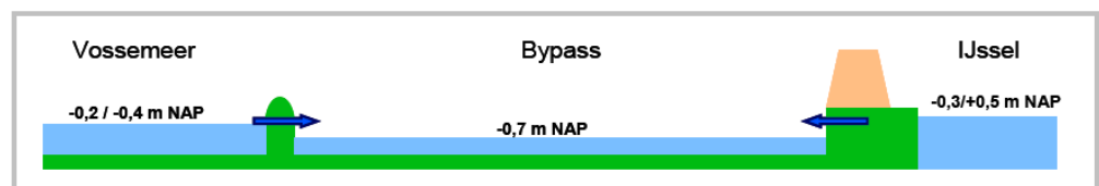
Figuur 6.22 Bypass onder dagelijkse omstandigheden met peilscheiding [DHV, 2009c]
