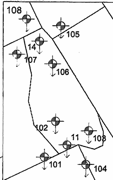
Nader onderzoek boring 11 en 14 Schaal: 1:250
