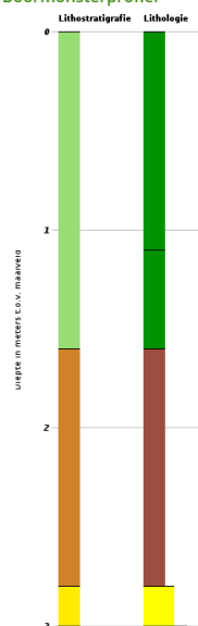
Boormonsterprofiel
